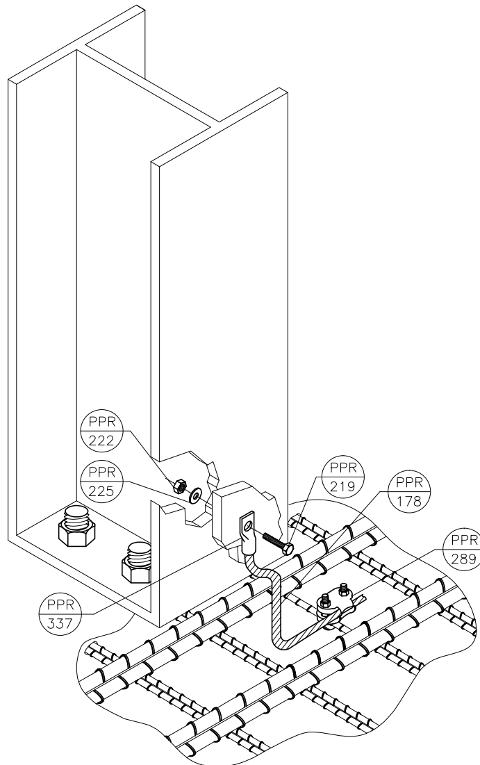
INTERLIGAÇÃO DE PILAR METÁLICO E BLOCO DE FUNDAÇÃO DETALHE A-1.06
