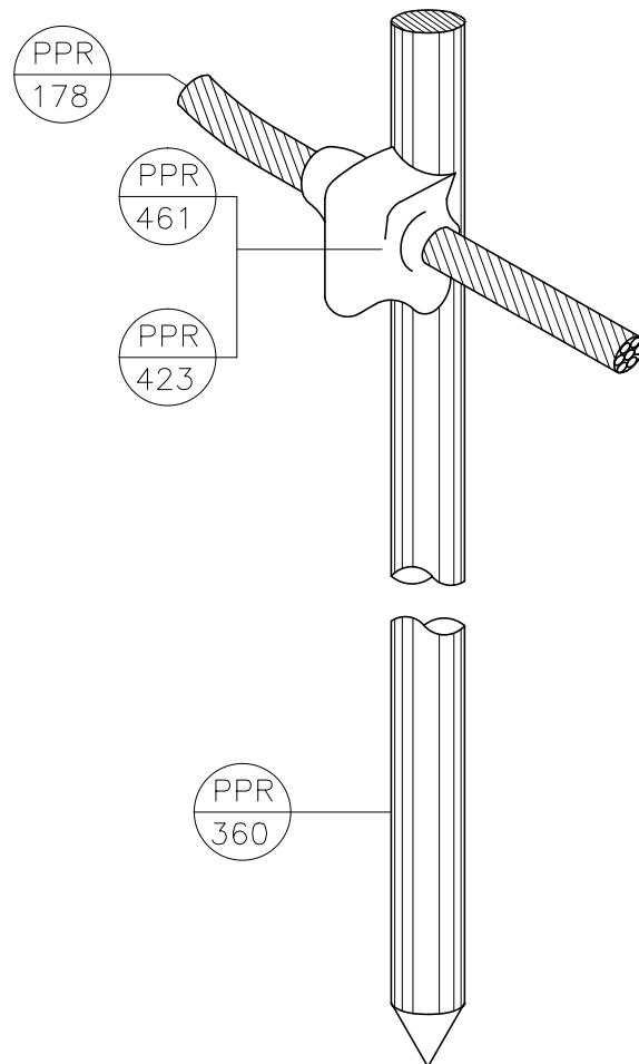
HASTE DE ATERRAMENTO 5/8" C/ CONEXÃO EXOTÉRMICA CABO PASSANTE DETALHE A-2.02
