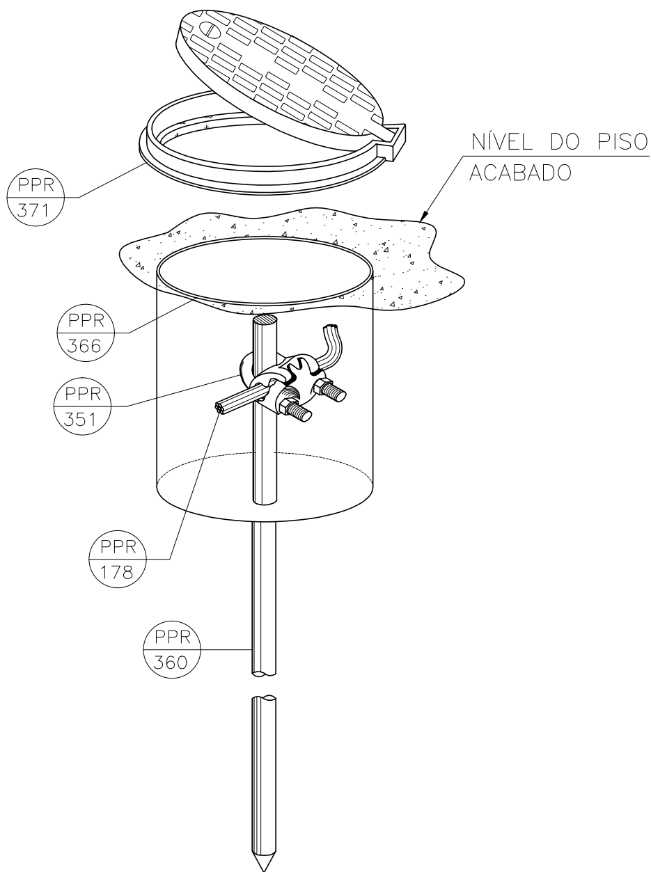
HASTE DE ATERRAMENTO 5/8" C/ CAIXA DE INSPEÇÃO REFORÇADA E GRAMPO CABO / HASTE DETALHE A-2.05
