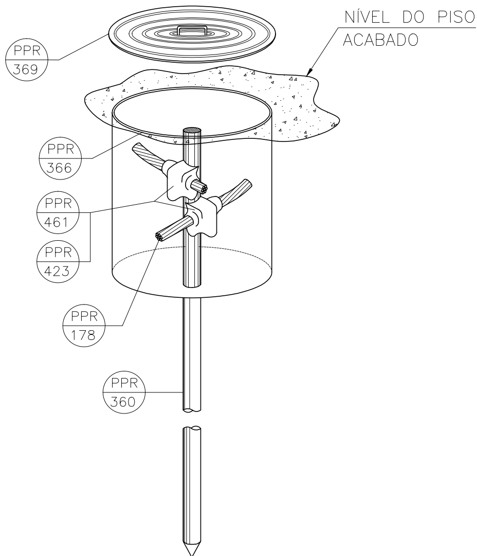
HASTE DE ATERRAMENTO 5/8" C/ CAIXA DE INSPEÇÃO Ø25cm C/ CONEXÃO EXOTÉRMICA DETALHE A-2.07
