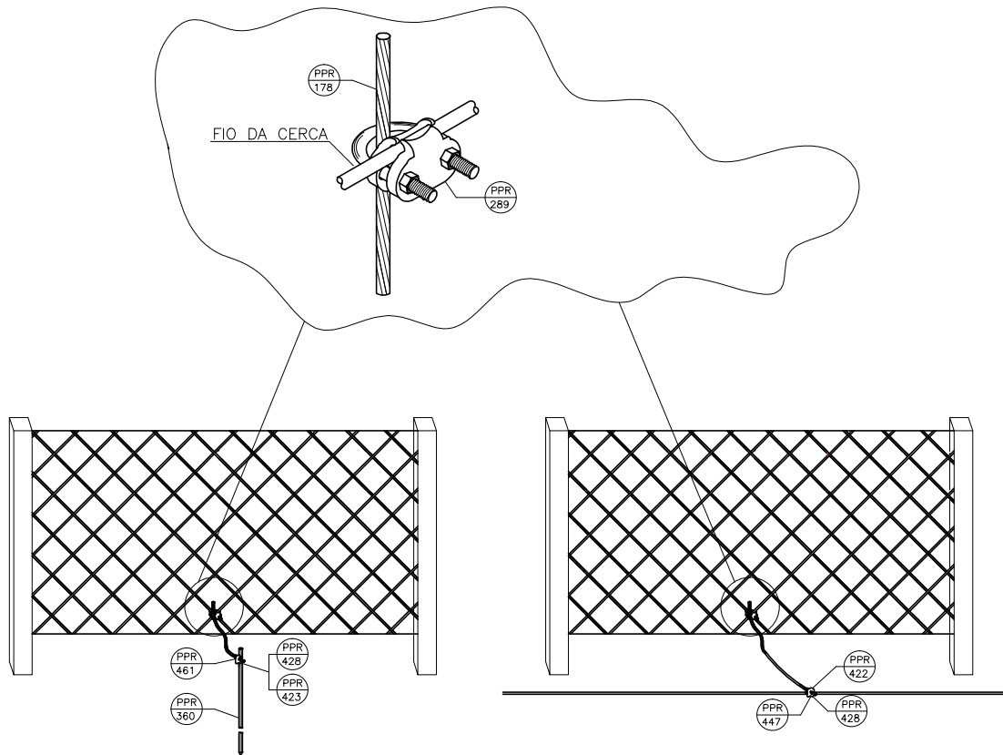
ATERRAMENTO DE TELA DETALHE A-1.02
