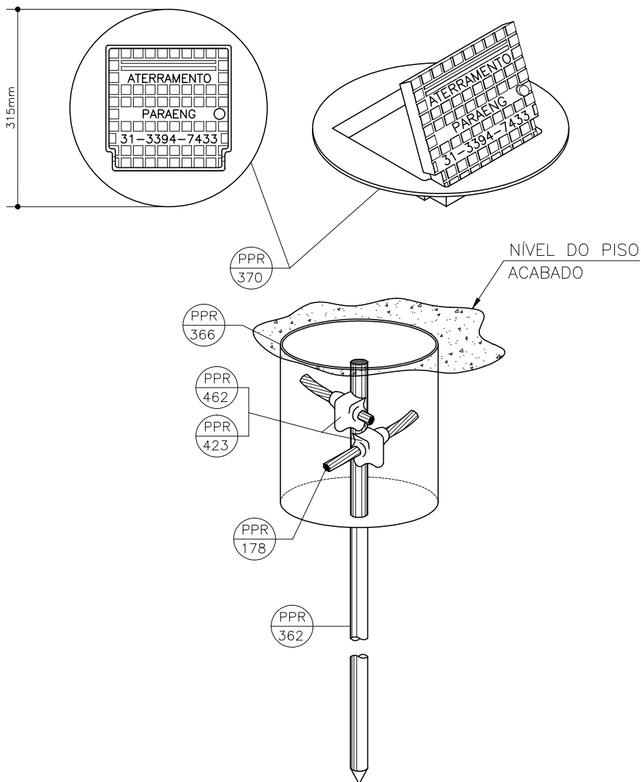
HASTE DE ATERRAMENTO 3/4" C/ CAIXA DE INSPEÇÃO ARTICULADA REFOÇADA E CONEXÃO EXOTÉRMICA DETALHE A-2.17
