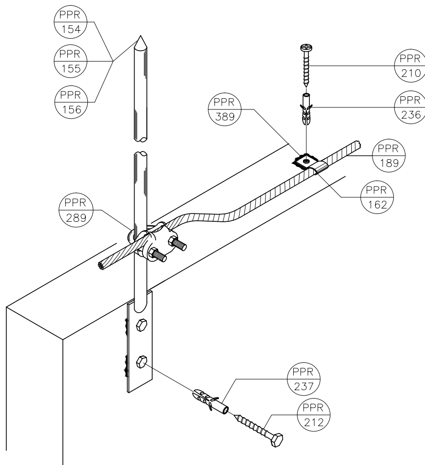
TERMINAL AÉREO CAPTOR C/ BASE VERTICAL DETALHE C-3.09
