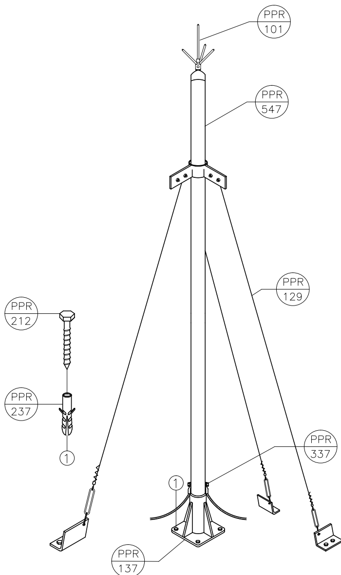
MASTRO CAPTOR COM ESTAIAMENTO RIGIDO H=9m DETALHE C-4.14
