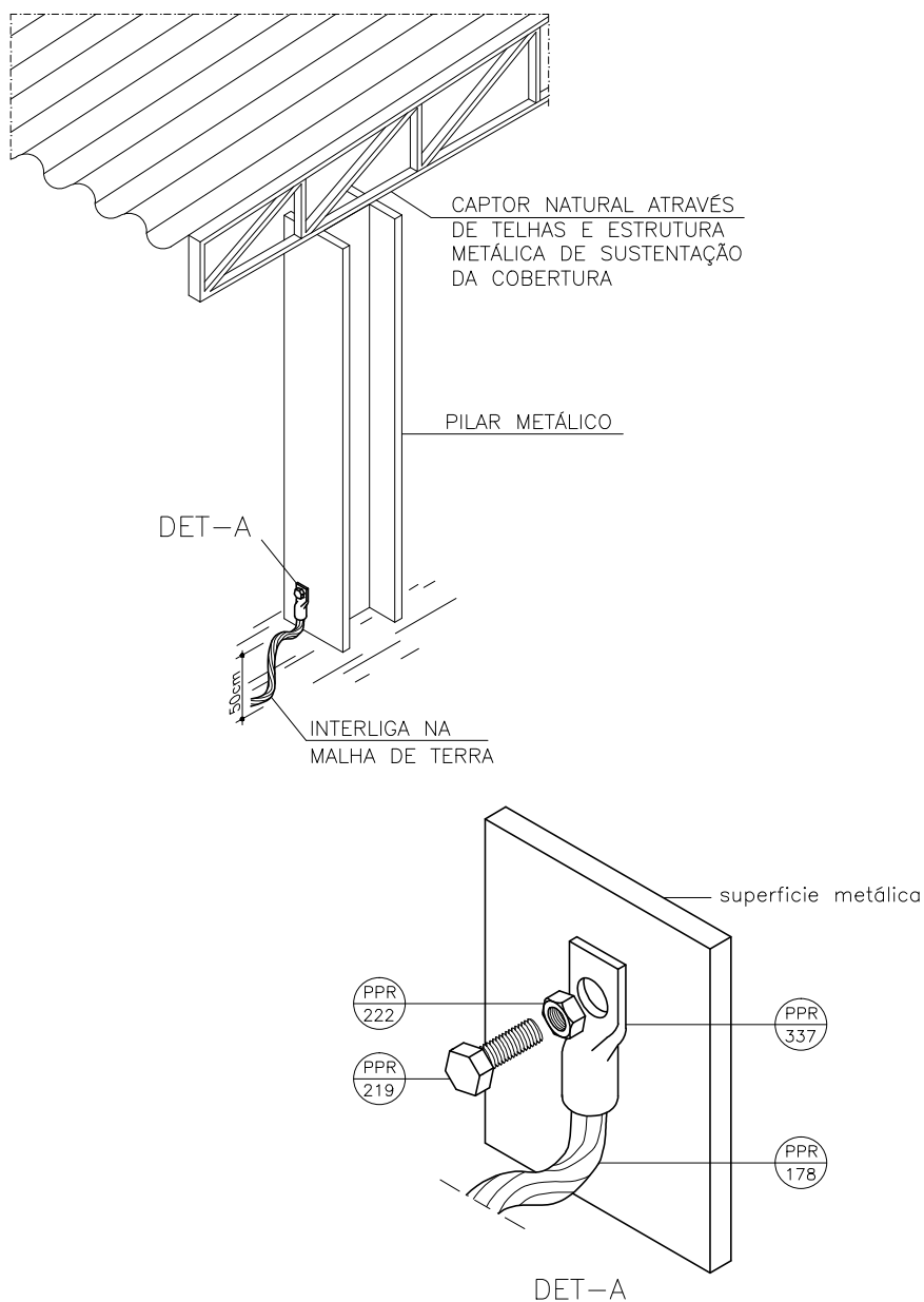
ESTRUTURA/PILAR METÁLICO USADO COMO DESCIDA NATURAL DETALHE D-3.02
