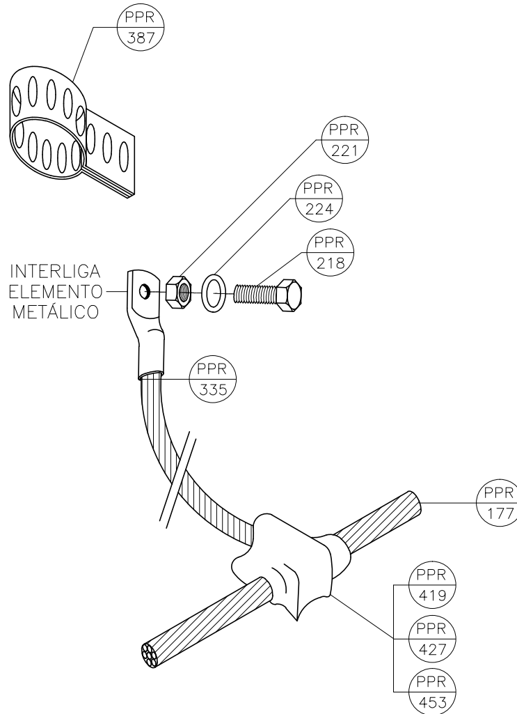
INTERLIGAÇÃO DE ELEMENTO METÁLICO Á PARTIR DE SOLDA EXOTÉRMICA EM CABO PASSANTE DETALHE EQ-1.09
